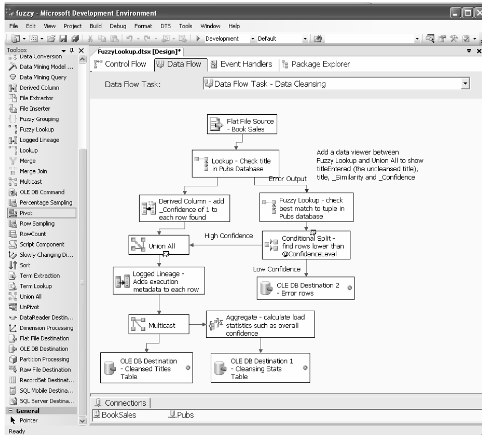
Figura 29.7 Carga de datos usando búsquedas difusas.
