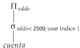
Figura 13.2 Plan de ejecución de una consulta.
