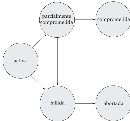
Figura 15.1 Diagrama de transición de estado de una transacción.
