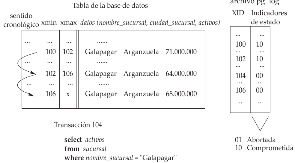
Figura 26.6 Las estructuras de datos de PostgreSQL empleadas para MVCC
